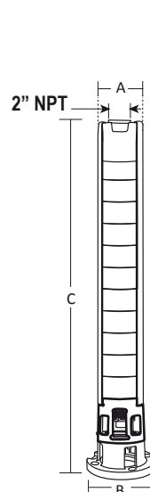
Acoplamiento NEMA 4"
