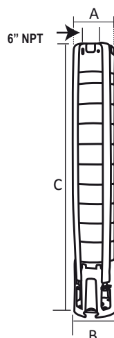
Acoplamiento NEMA 8"
