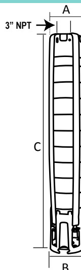
Acoplamiento NEMA 6"
